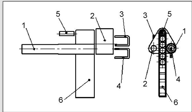
Рис.1: 1 — ствол, 2 — барабан, 3 — экстрактор, 4 — ударный механизм, 5 — толкатель, 6 — магазин.
