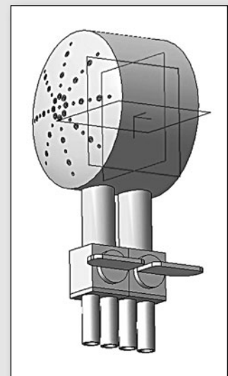
Рис.2: 1 — основной смеситель, 2 — дополнительный смеситель, 3 — основная головка, 4 — дополнительная головка, 5 — отверстия, 6 — патрубки.
