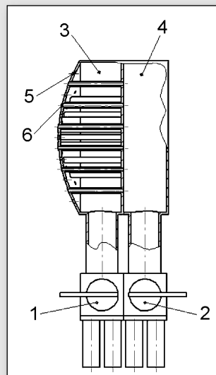
Рис.2: 1 — основной смеситель, 2 — дополнительный смеситель, 3 — основная головка, 4 — дополнительная головка, 5 — отверстия, 6 — патрубки.
