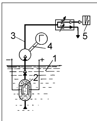
Рис.1. Электрогидравлическая станция Юткиных.
