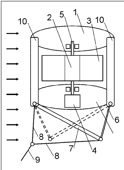
Гидроэлектрическая установка.
